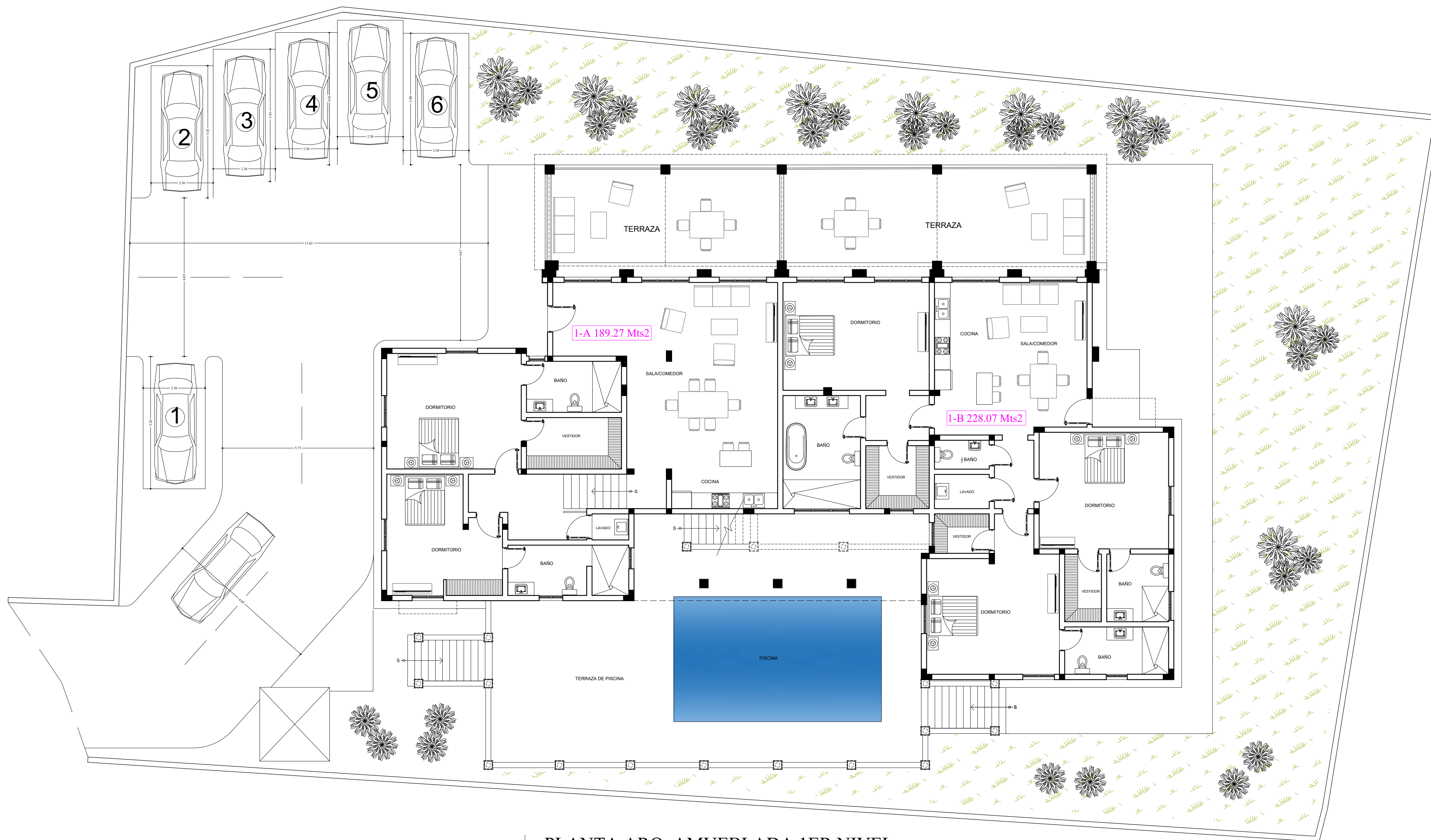
PLANTA ARQ. AMUEBLADA 1ER NIVEL EL CASTILLO Esc. 1:100
